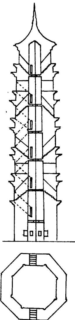
大胜宝塔结构示意图
